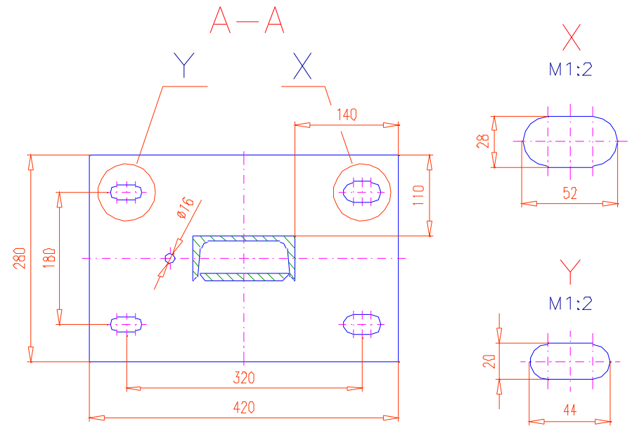
PROVEDENÍ SLOUPKU S PODÉLNÝM SKLONEM PATNÍ DESKY
