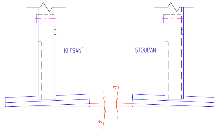
PROVEDENÍ SLOUPKU S PODÉLNÝM SKLONEM PATNÍ DESKY
