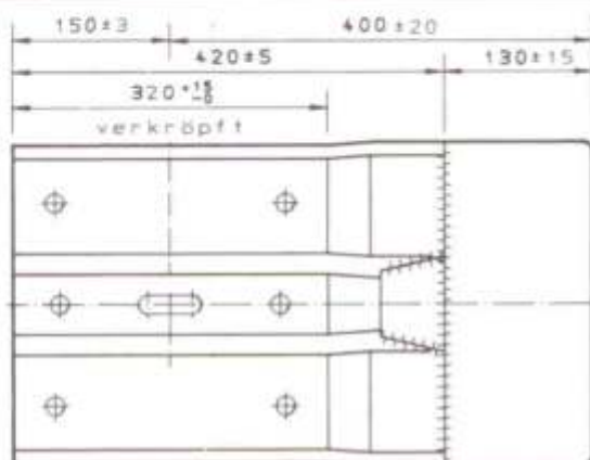
Teil Nr. 12.11 Kopfstück mit Tropflöchern
