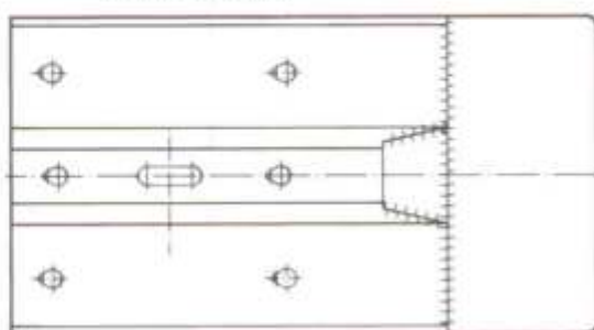
Teil Nr. 12.11 Kopfstück mit Tropflöchern
