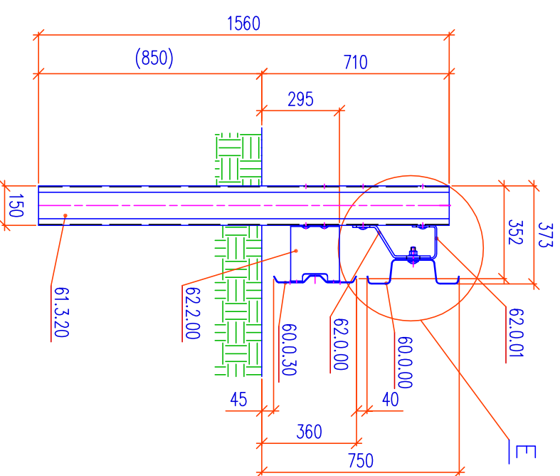
CELKOVÉ USPOŘADÁNÍ M 1:100
