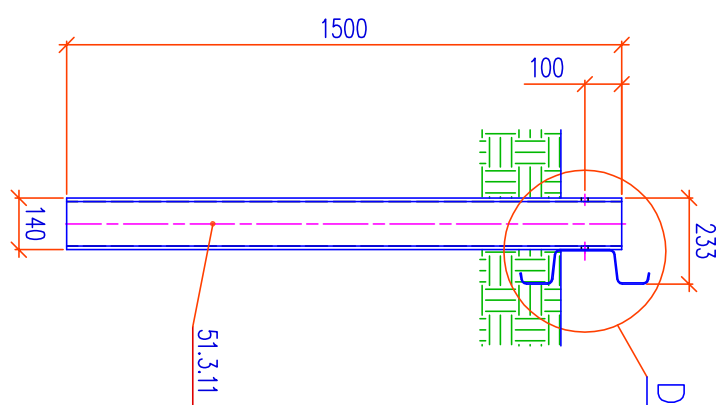
ŘEZ A-A M 1:20
